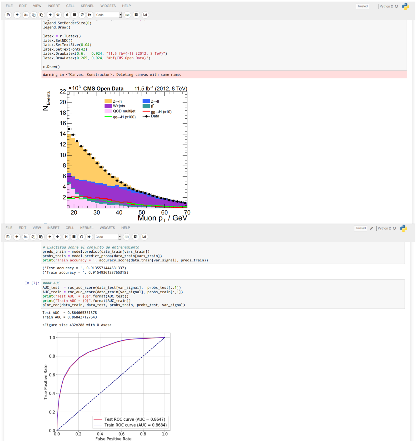
Figura 1: Visualización de los cuadernos de Jupyter dados a los estudiantes para realizar el proyecto.
