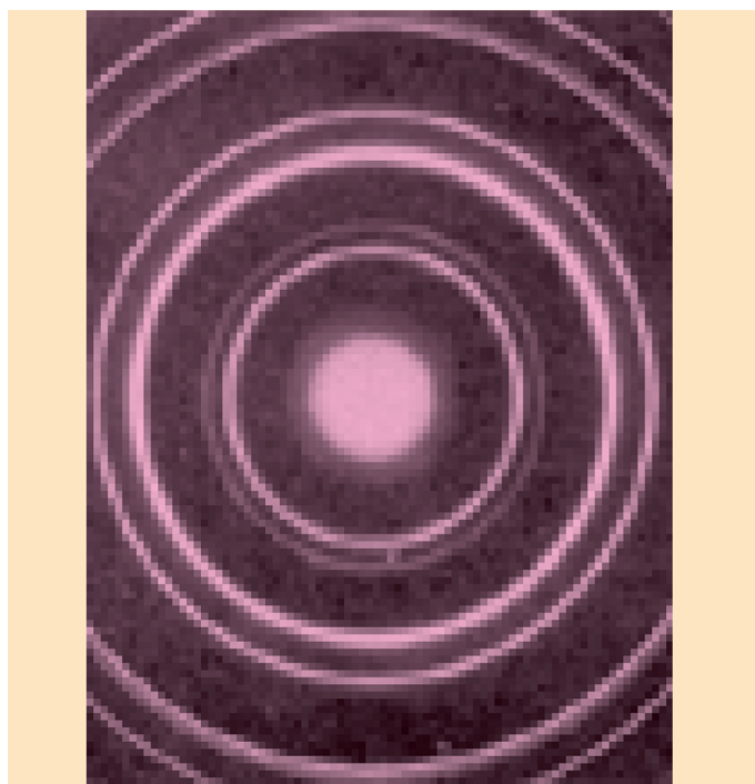
Figura 2. Imagen de difracción producida por electrones al atravesar una red de átomos (oro cristalino)
