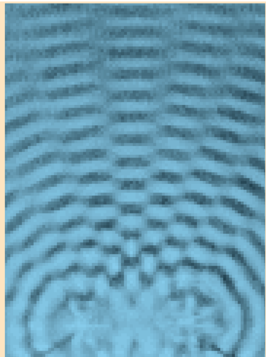
Figura 1. Fotografía de la figura de interferencia entre dos ondas, en una superficie de agua
